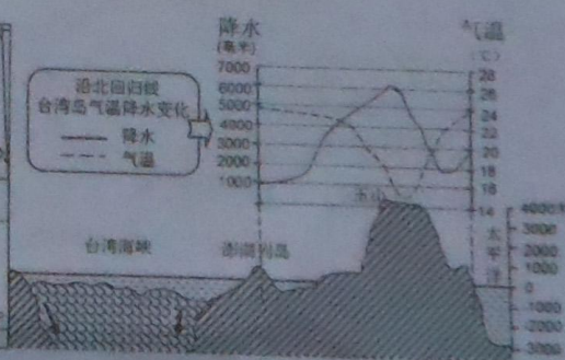
沿北回归线地形剖面图
